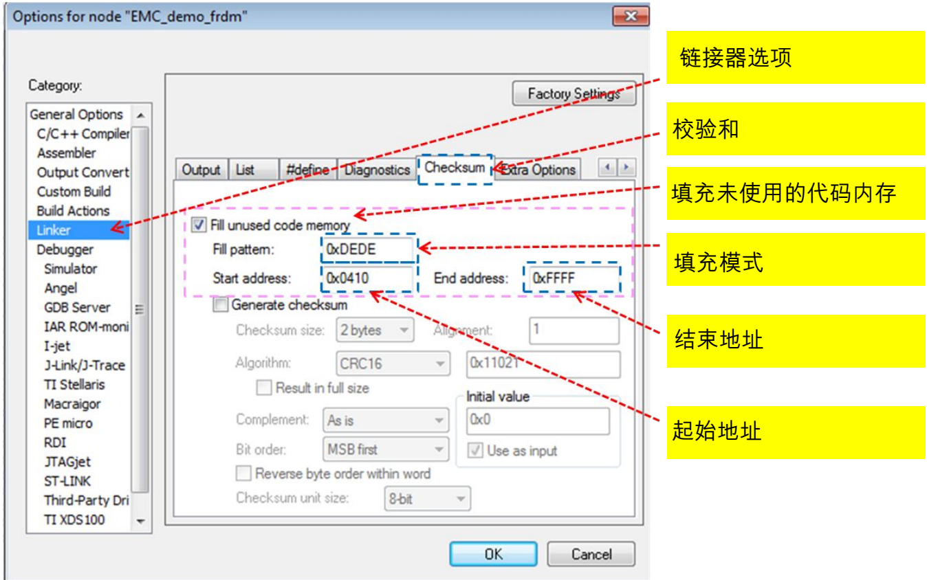
图 7. IAR 链接器选项
